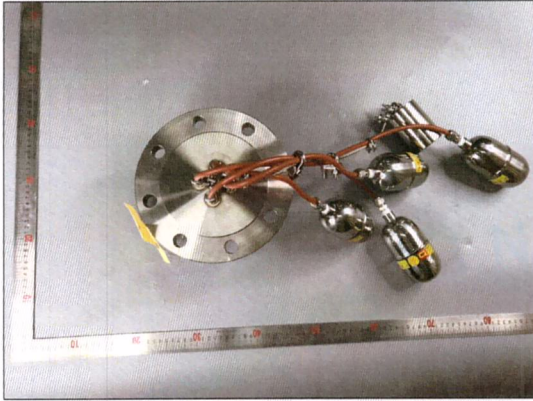
[그림 1: 시험품]
